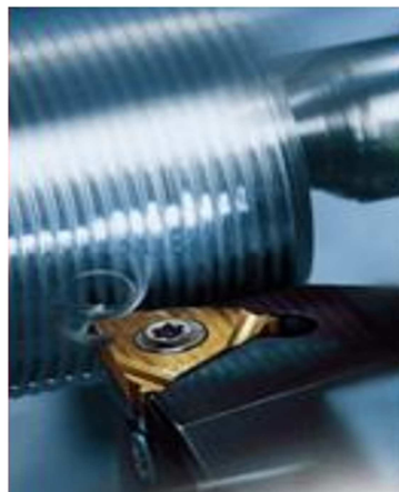
FIGURA 08 – Processo de corte de roscas.
